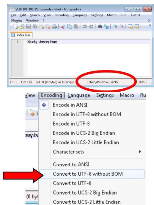
Εικόνα 2 - Μετατροπή κωδικοποίησης με το notepad++
